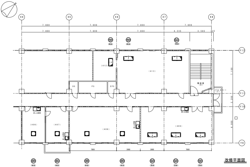
撤去平面図
