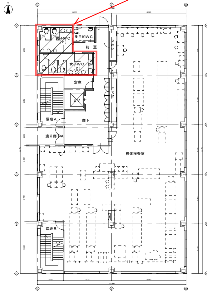
臨床検査棟 2 階平面図（改修後） S = 1 / 2 0 0
