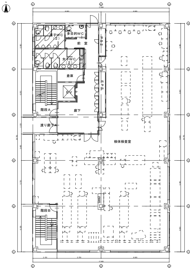
臨床検査棟 2 階平面図（改修前） S = 1 / 2 0 0
