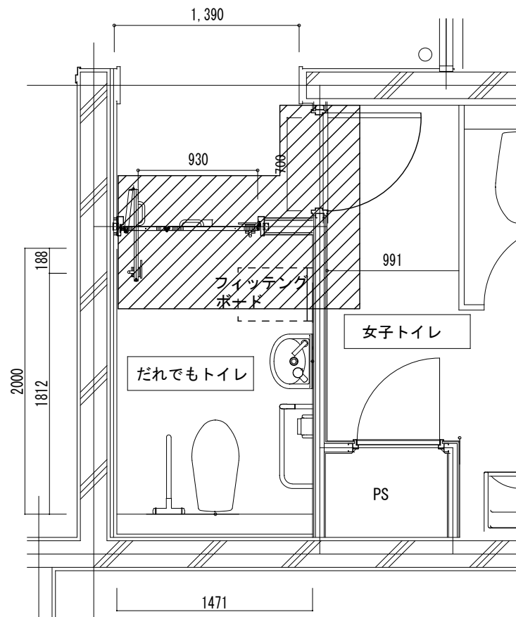
川内講義棟 A 改修トイレ平面図
