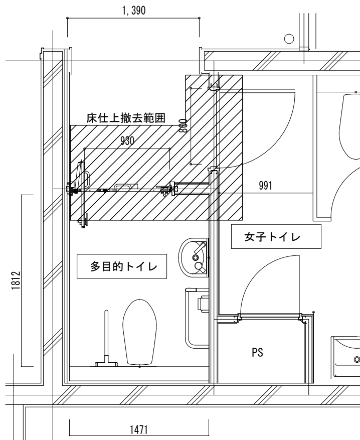
川内講義棟 A 既存トイレ平面図
