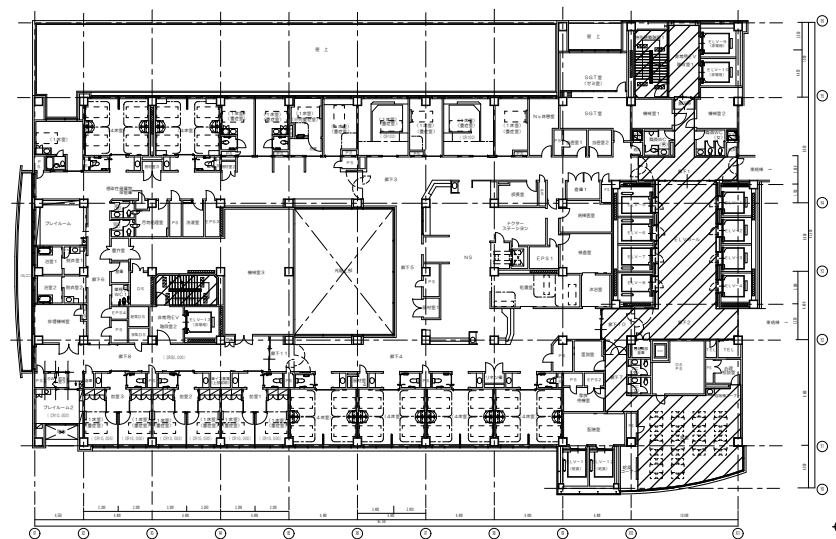
西病棟 5階 平面図
