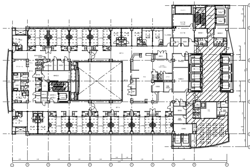
西病棟 7～12階, 14～16階 平面図
