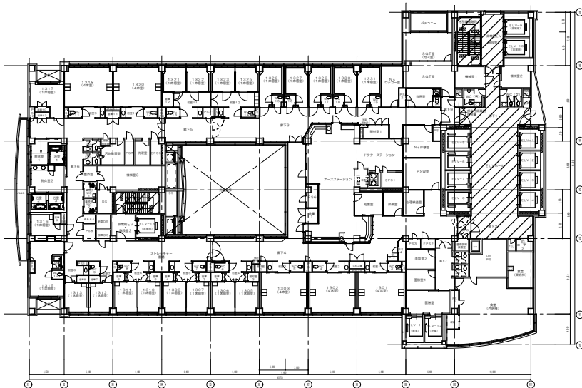
西病棟 13階 平面図
