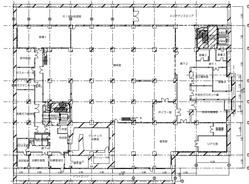
西病棟 地下2階 平面図
