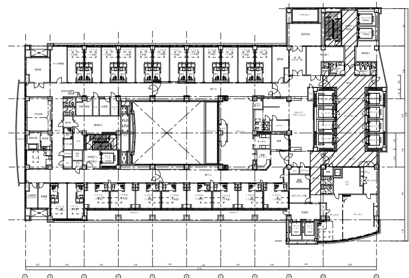
西病棟 17階 平面図
