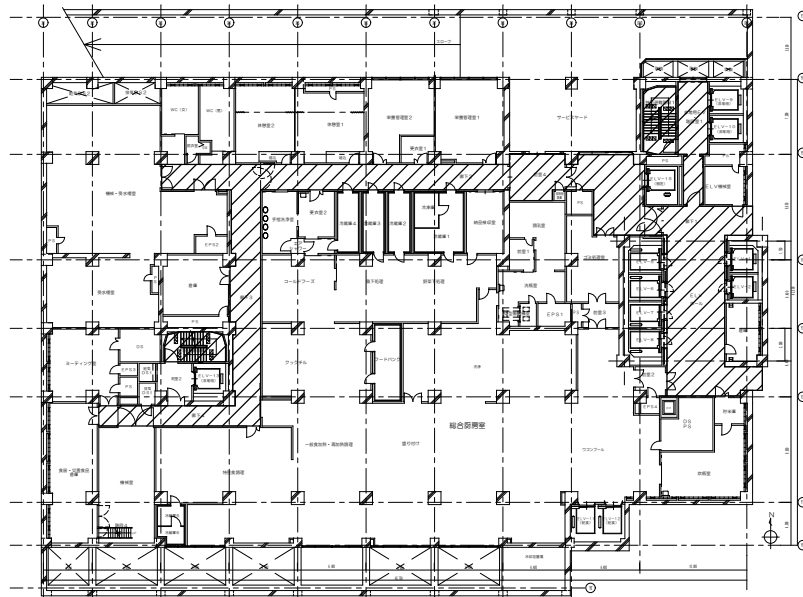
西病棟 地下1階 平面図
