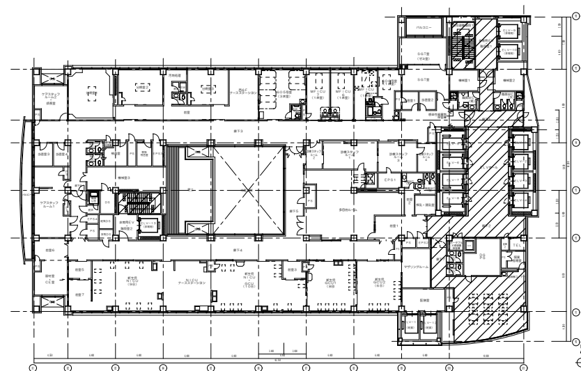
西病棟 6階 平面図
