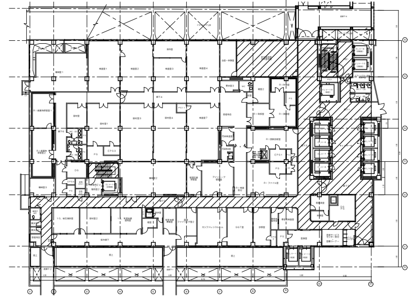
西病棟 1階 平面図
