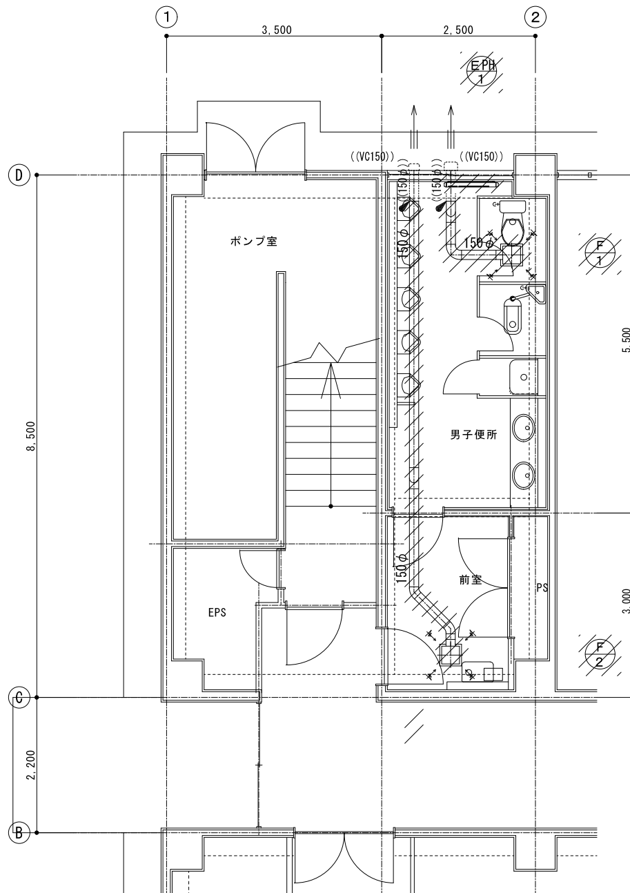
1階詳細図 S=1/60
