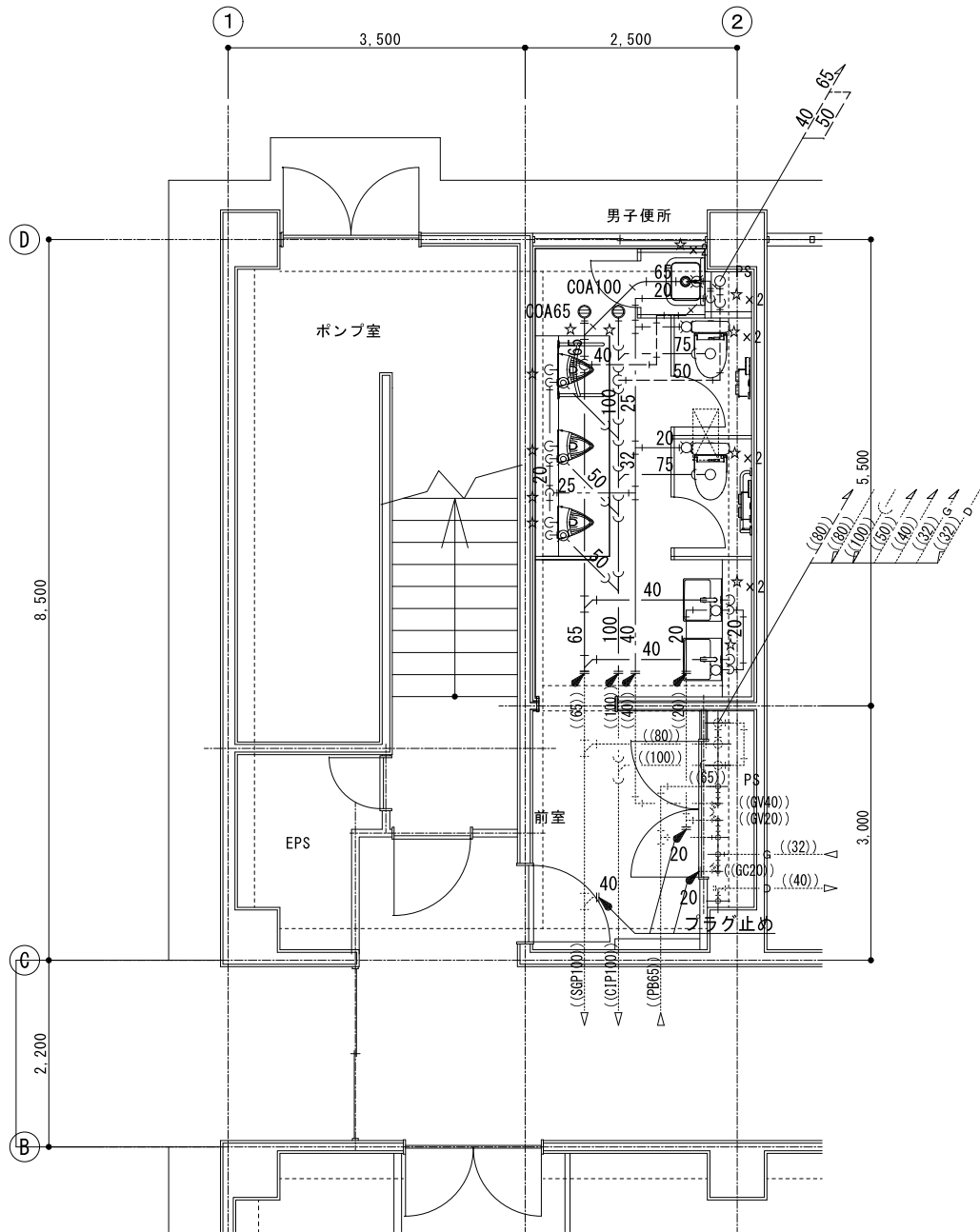
1階詳細図 S=1/60
