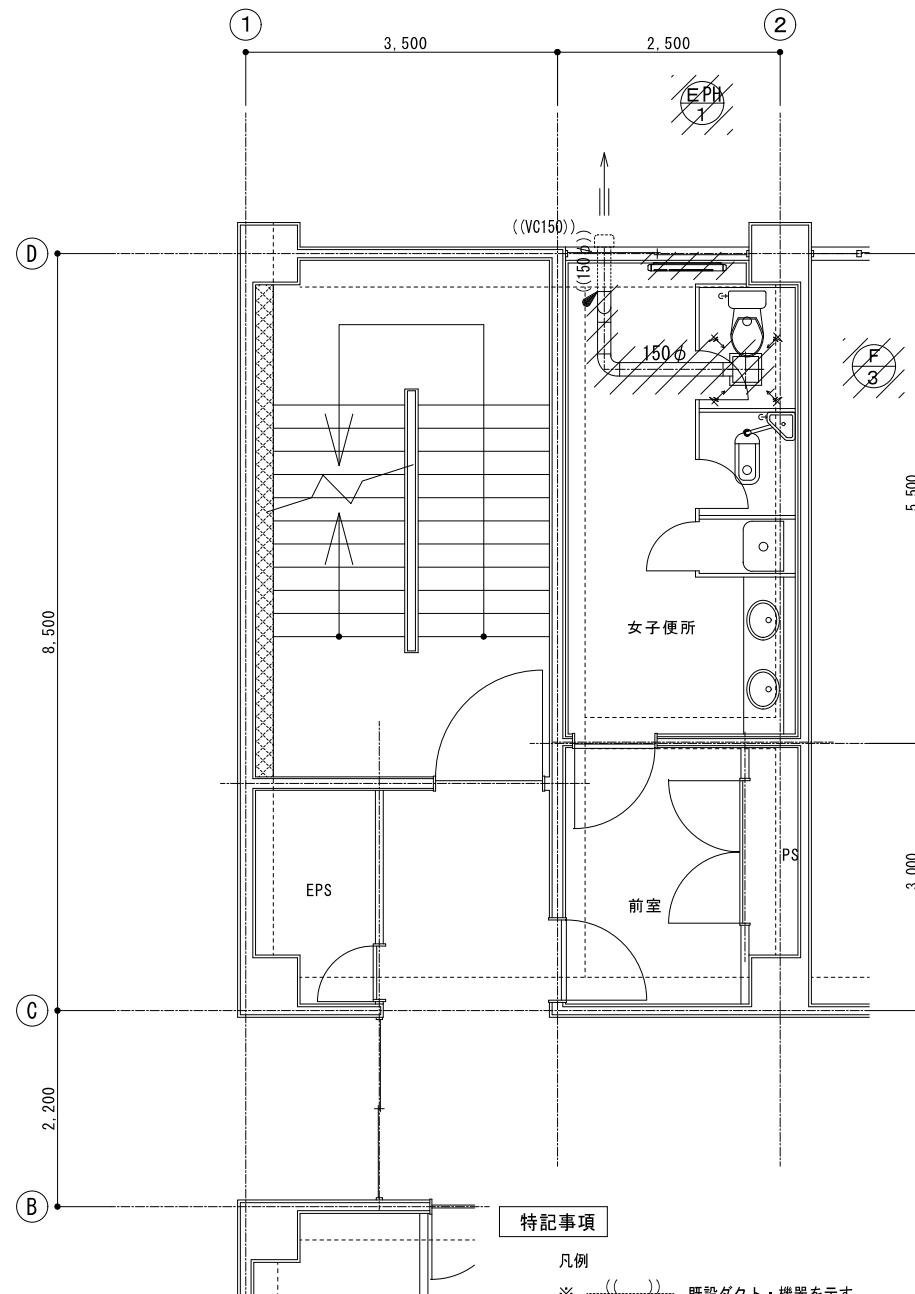
2階詳細図 S=1/60
