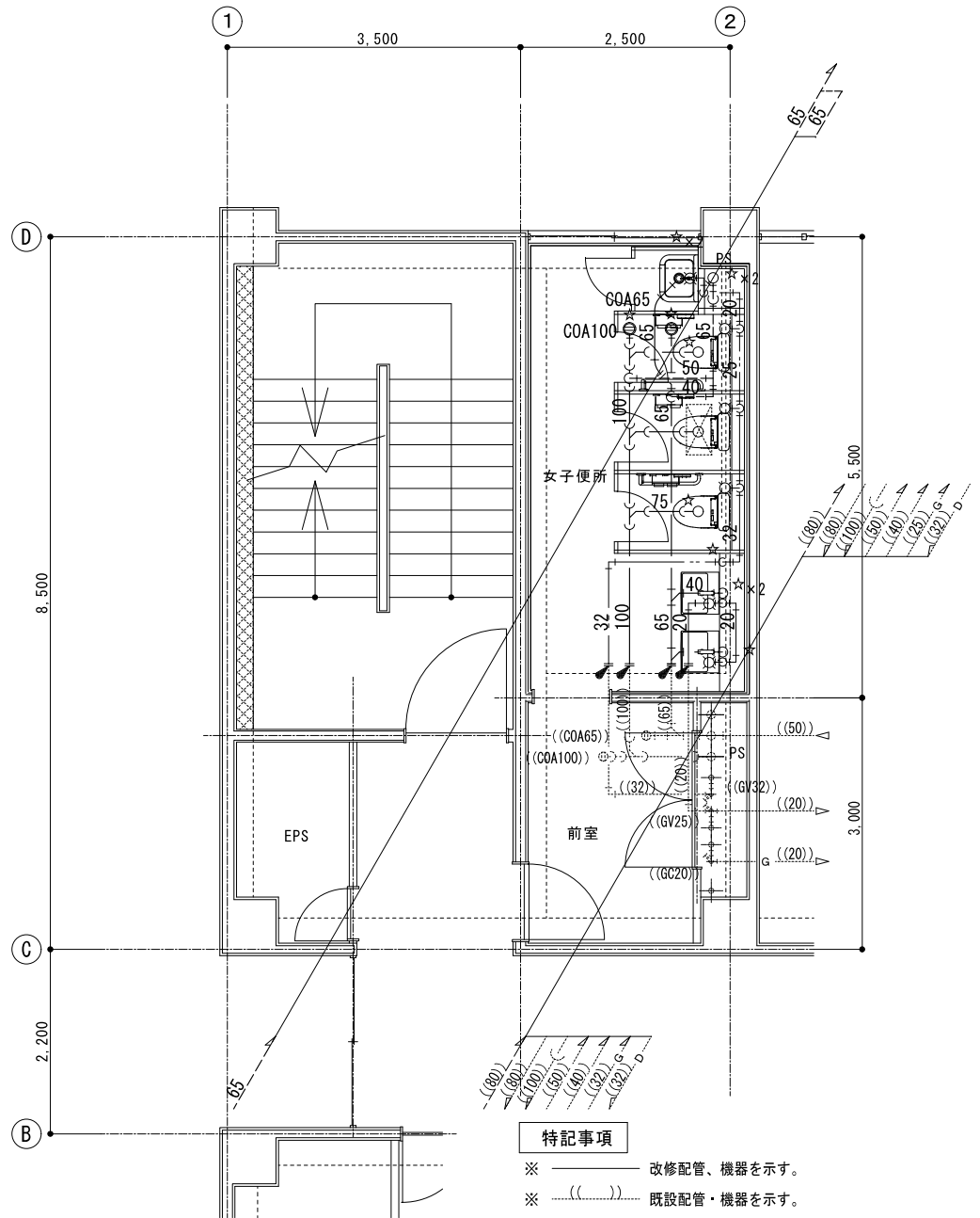
2階詳細図 S=1/60
