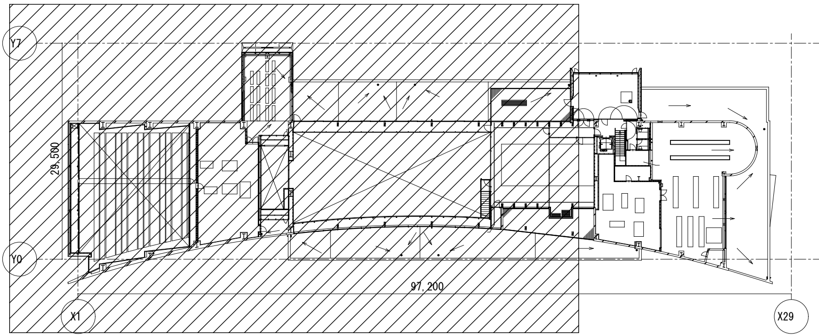
中央棟 4階平面図 キープラン
