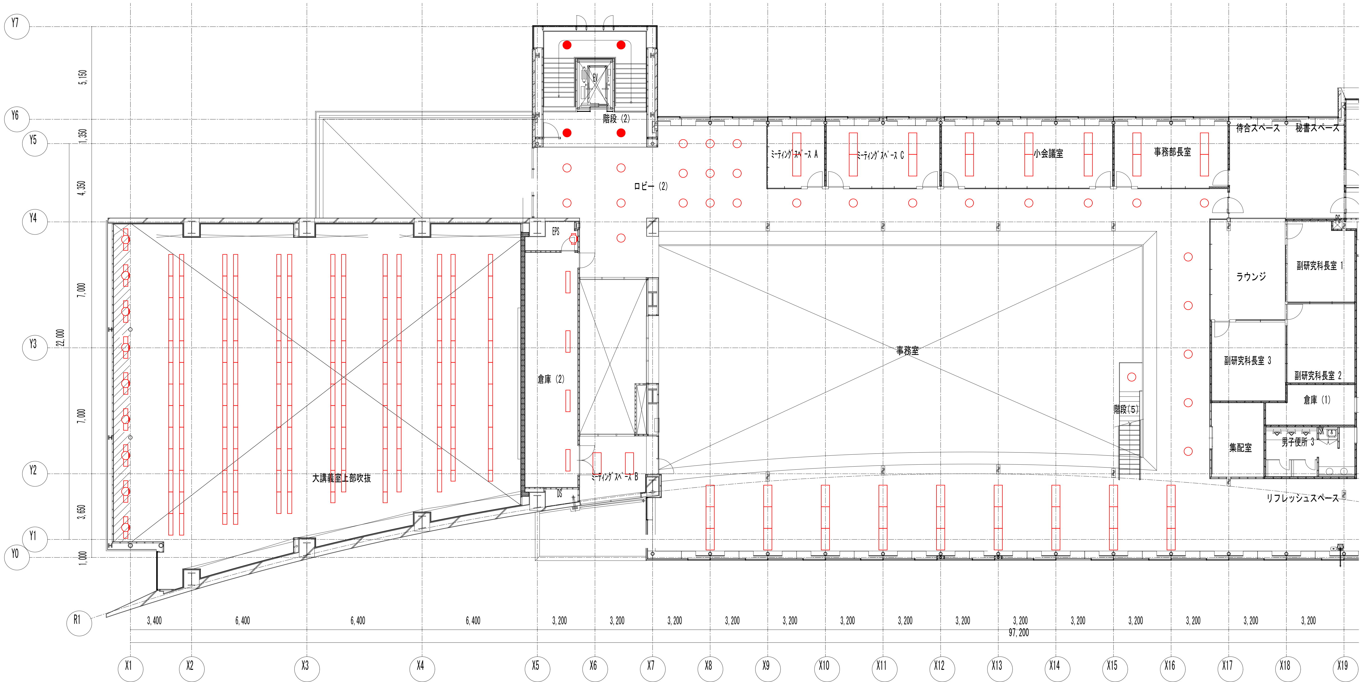
中央棟 3階平面図（1）
