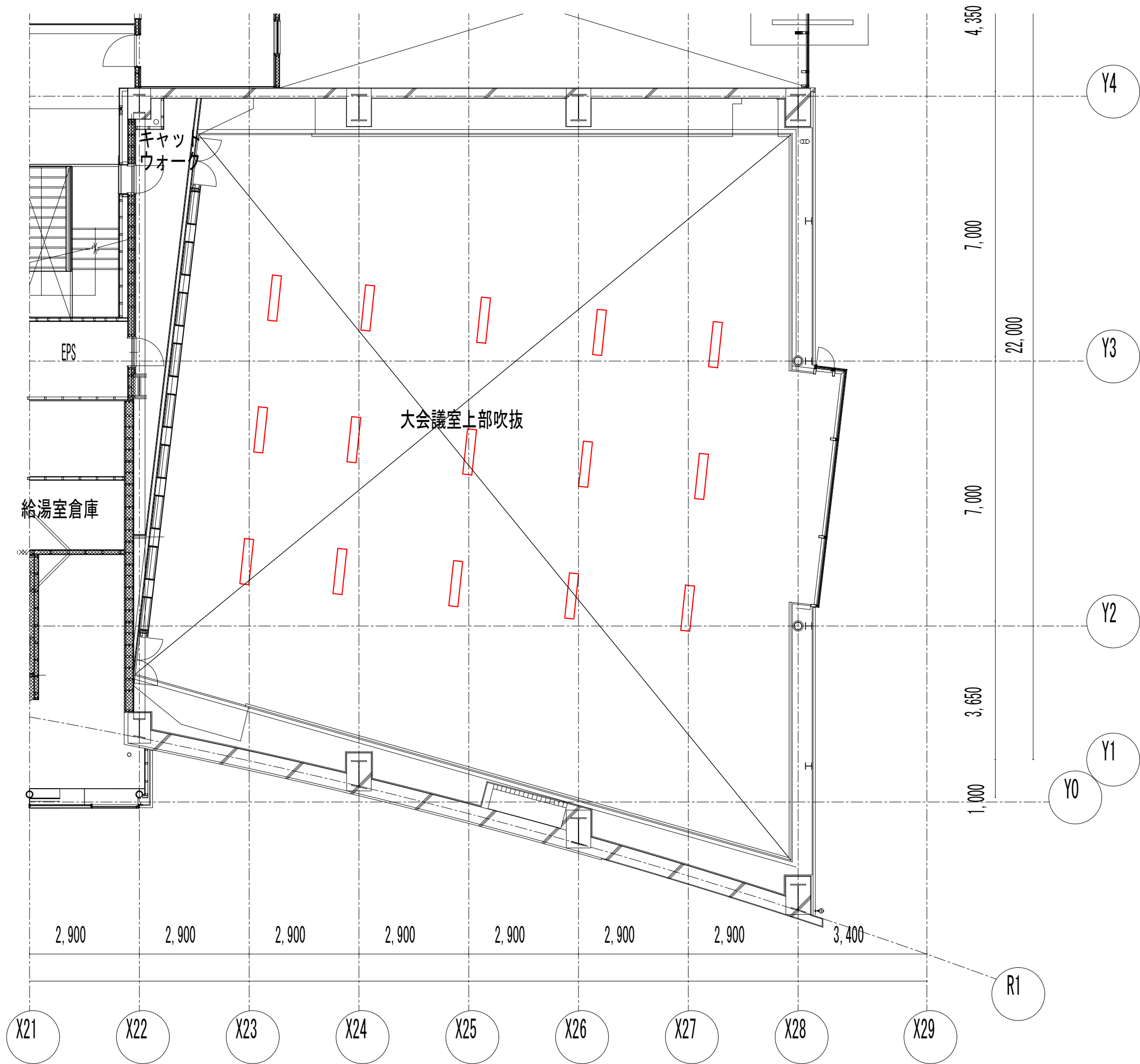
中央棟 3階平面図（3） 大会議室上部
