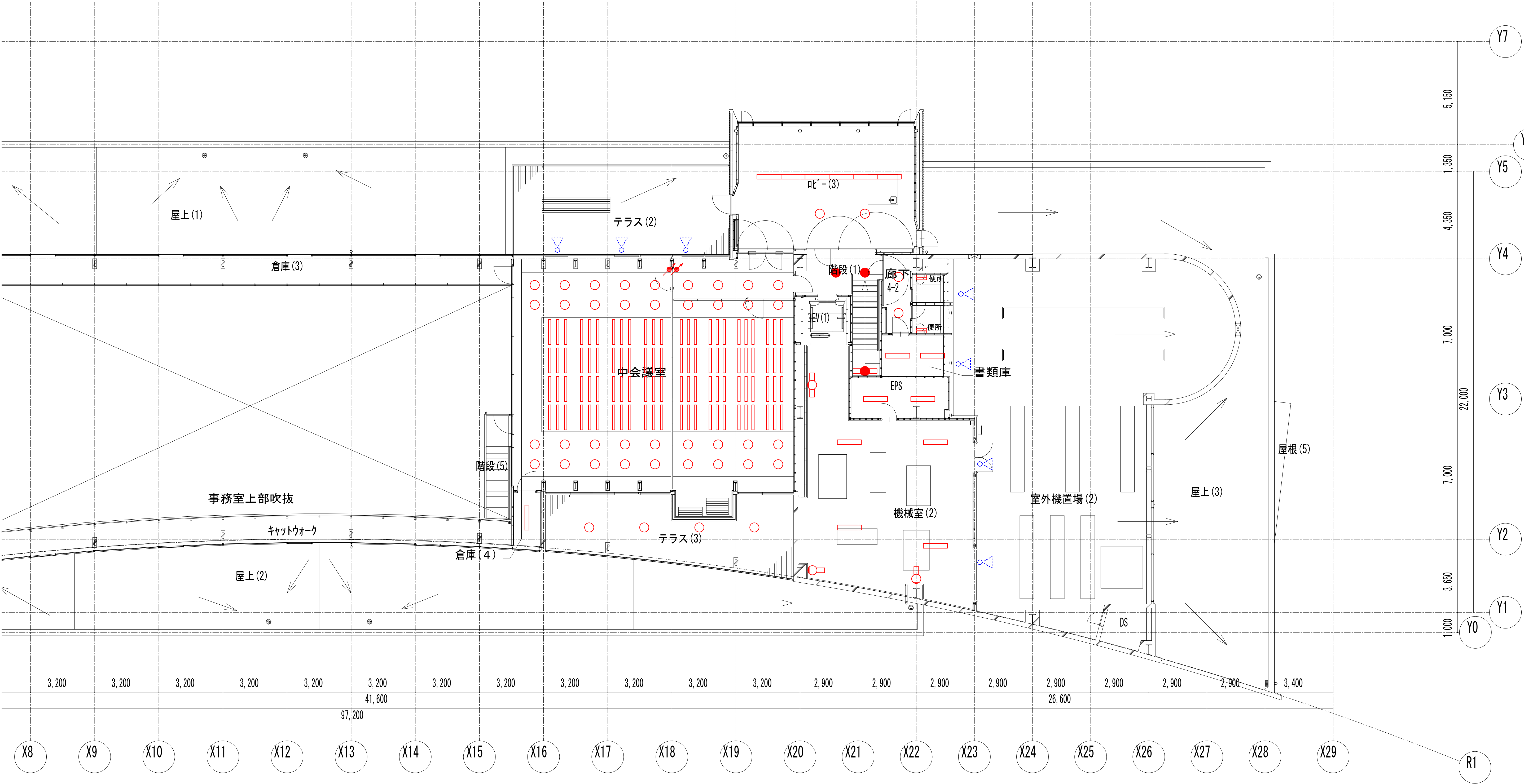
中央棟 4階平面図（2）
