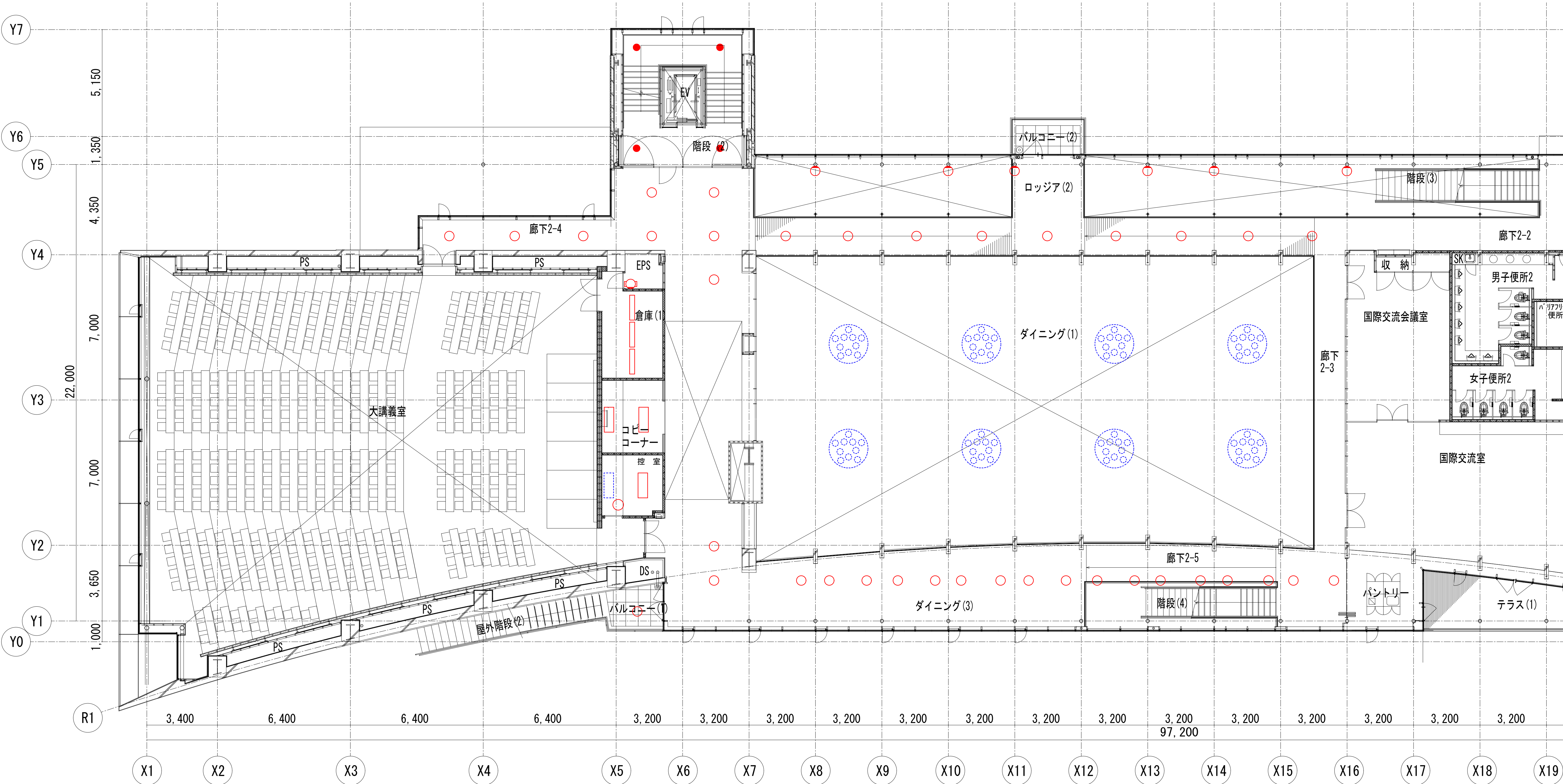
中央棟 2階平面図（1）
