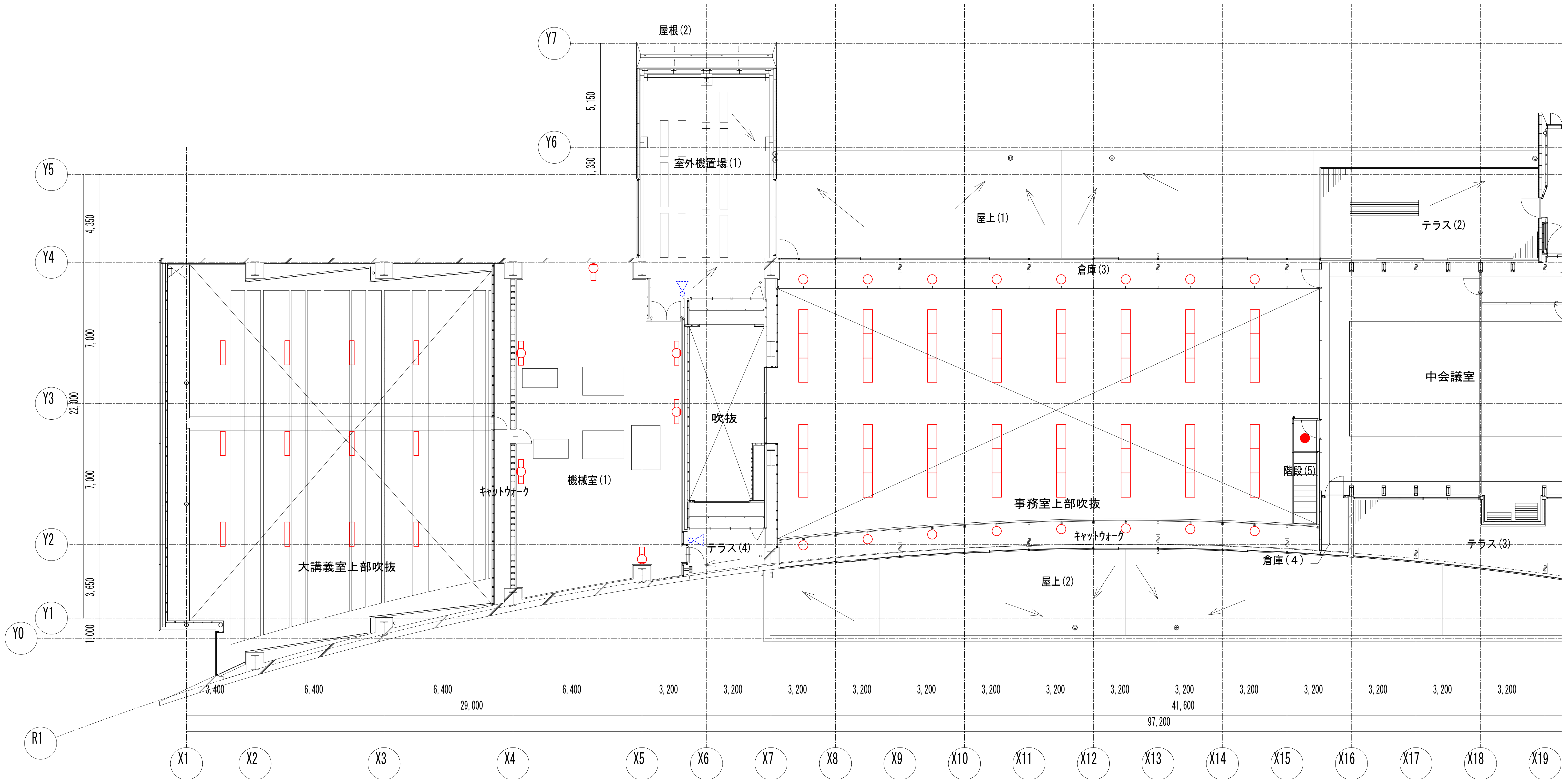
中央棟 4階平面図 (1)
