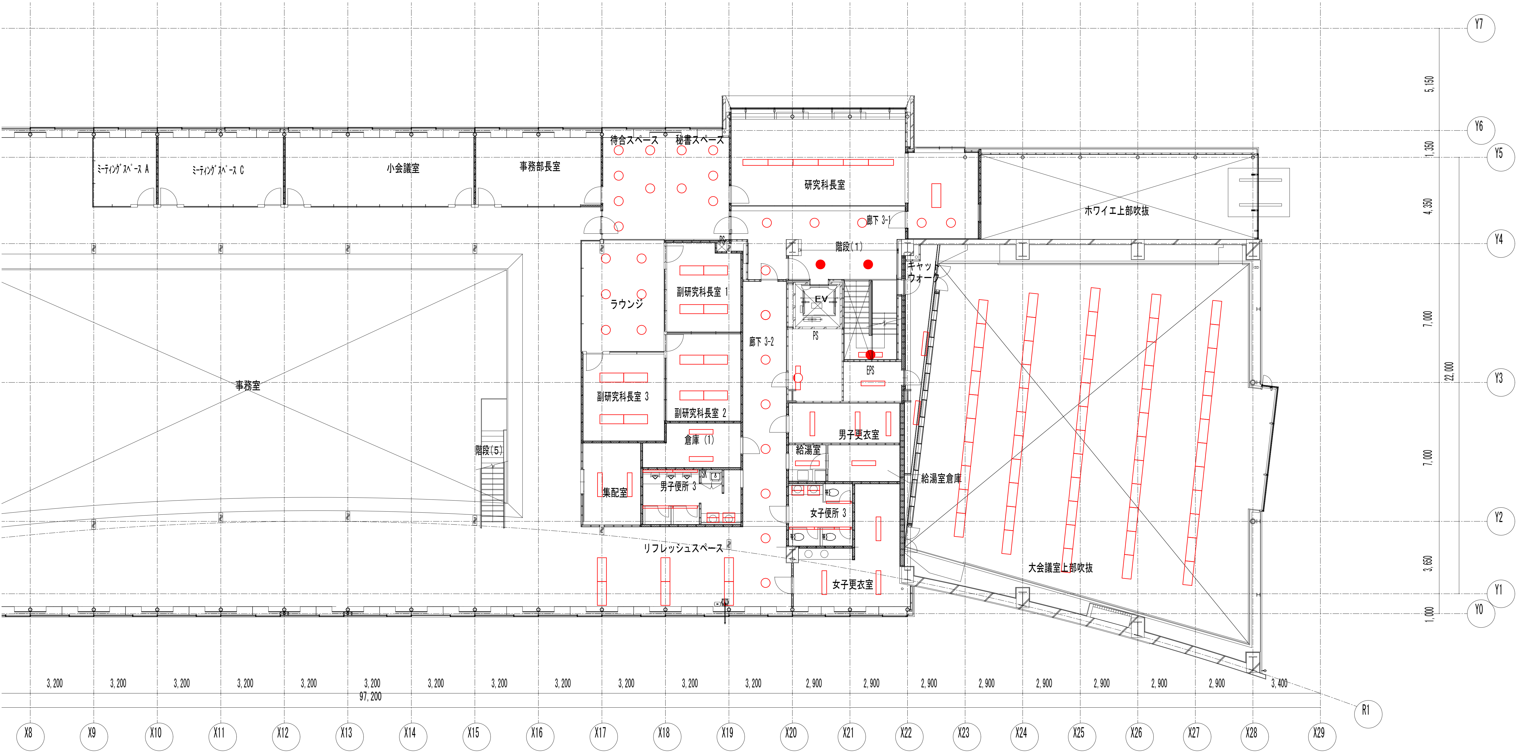
中央棟 3階平面図（2）
