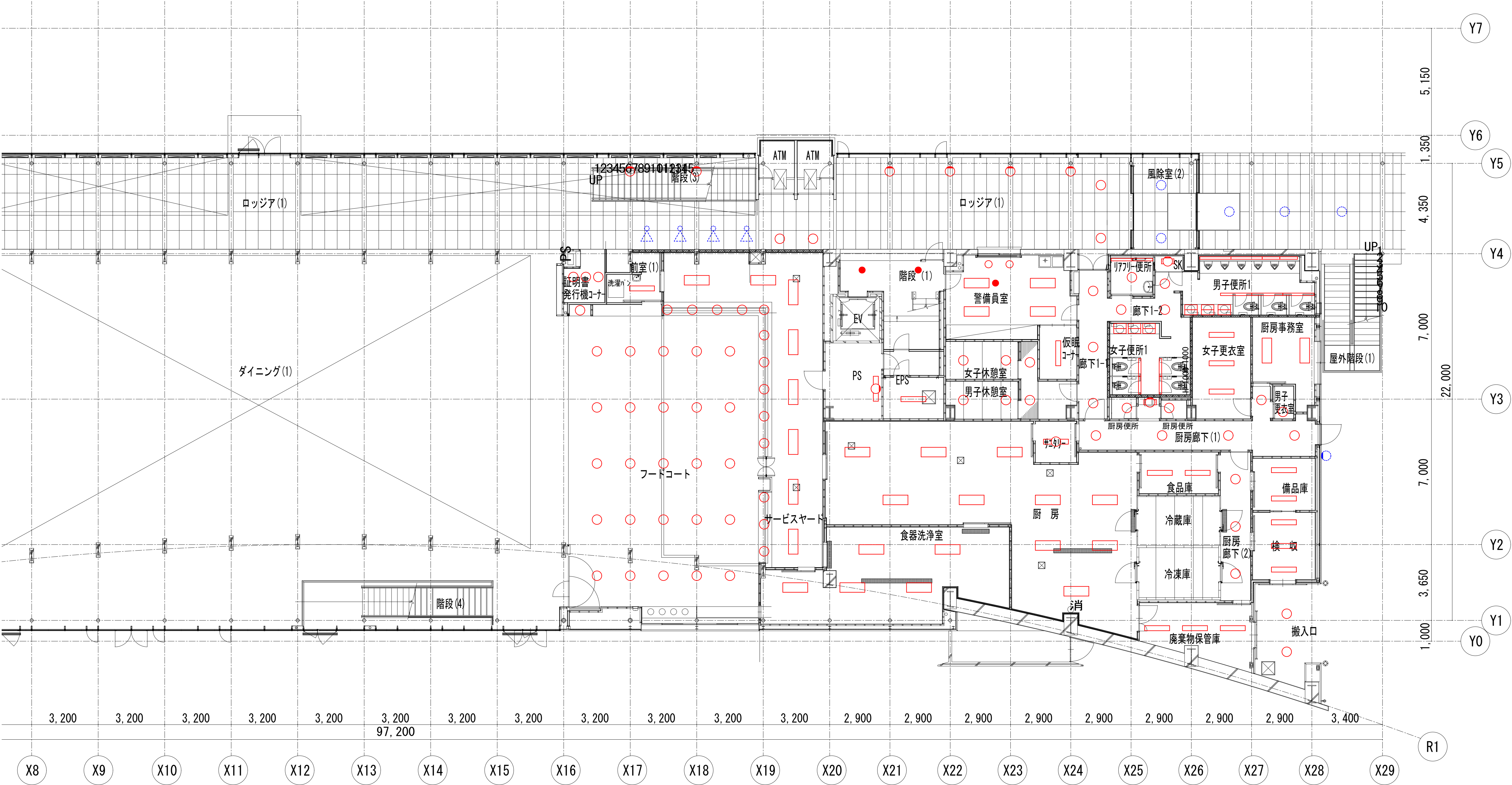
中央棟 1階平面図 (2)
