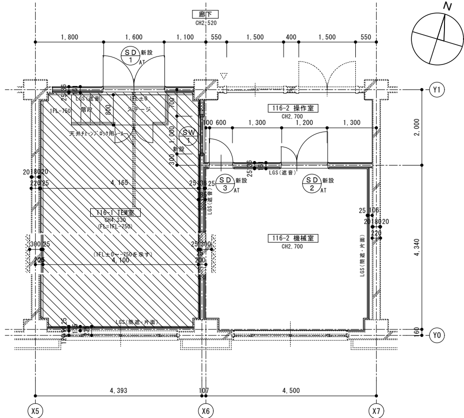
改修平面図 S=1/100
