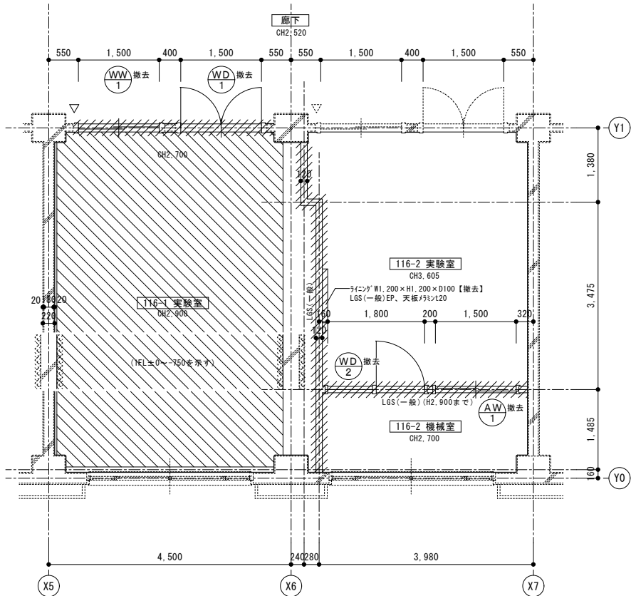
既存平面図 S=1/100
