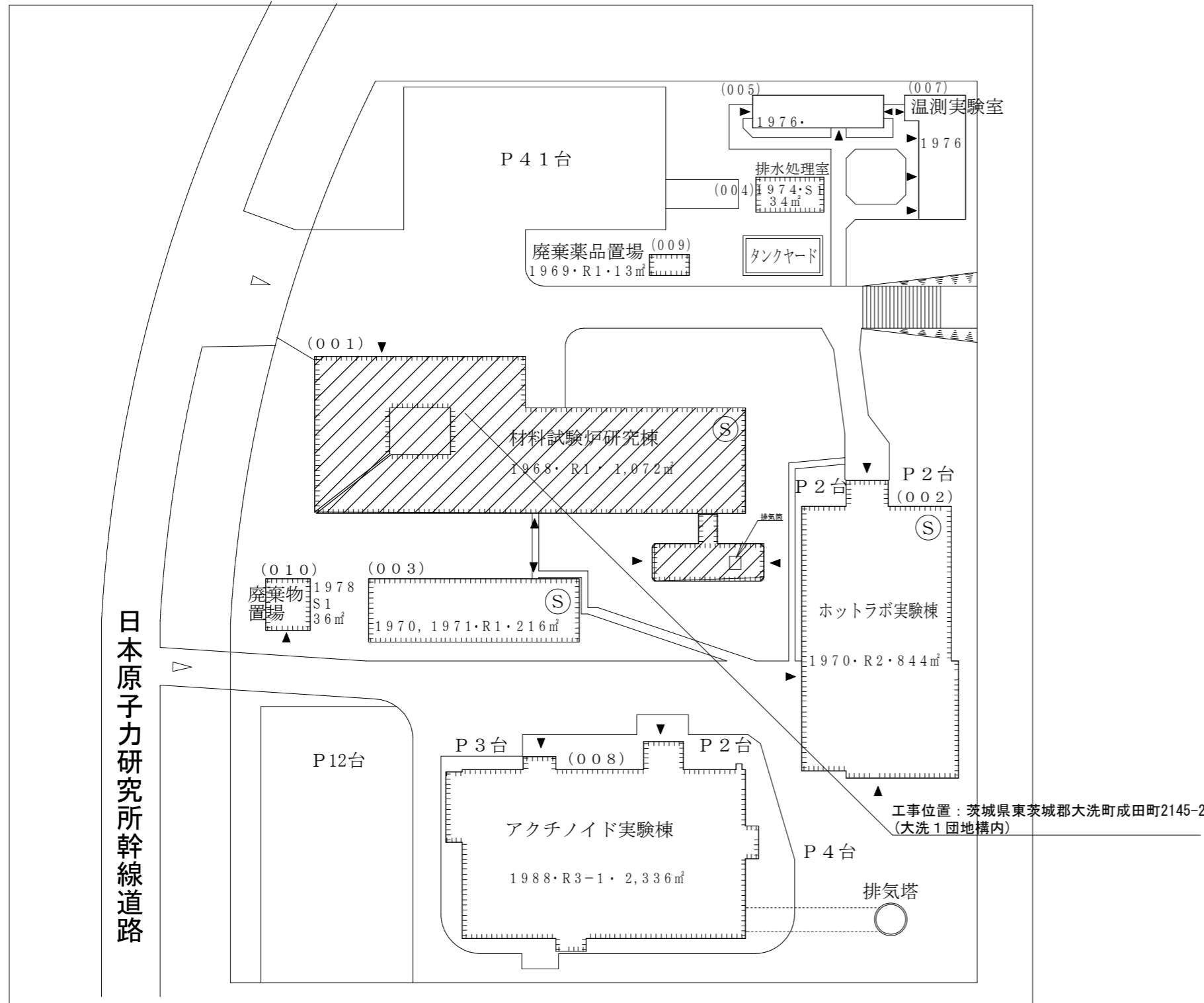
大洗1団地 配置図 S-NS
