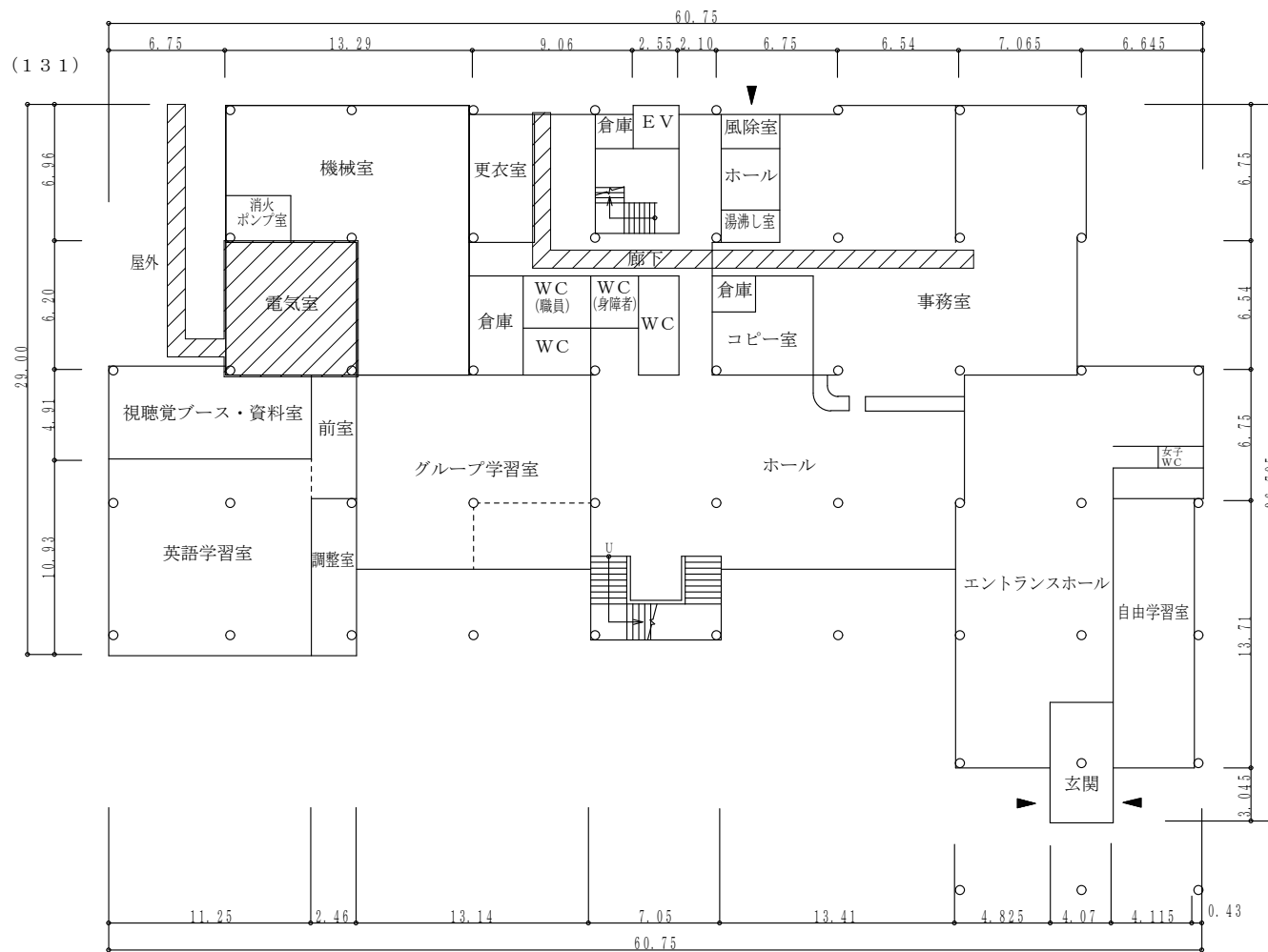
1階 平面図 1,507 m 2 S=1/400
