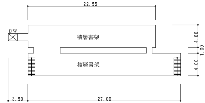
1階, 中2階平面図 199㎡ S=1/400
