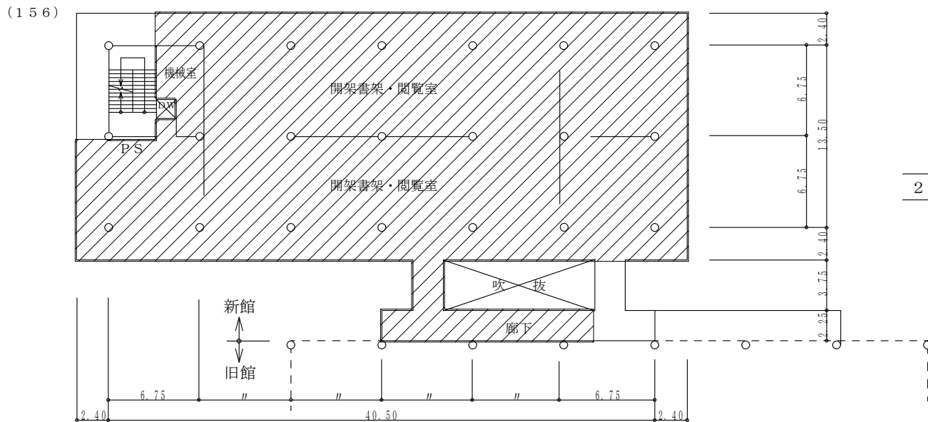
附属図書館工学分館（新館）平面図
