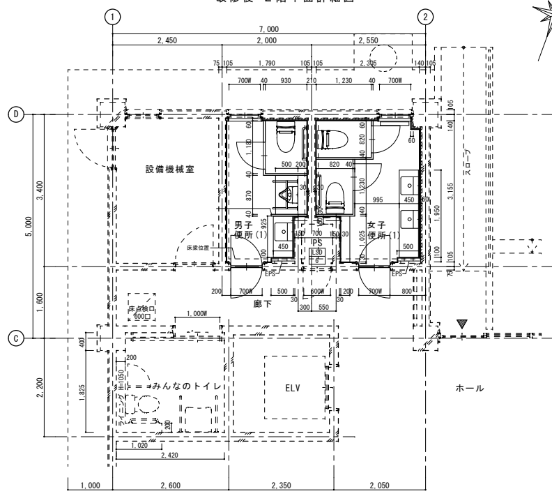
改修後 1階平面詳細図
