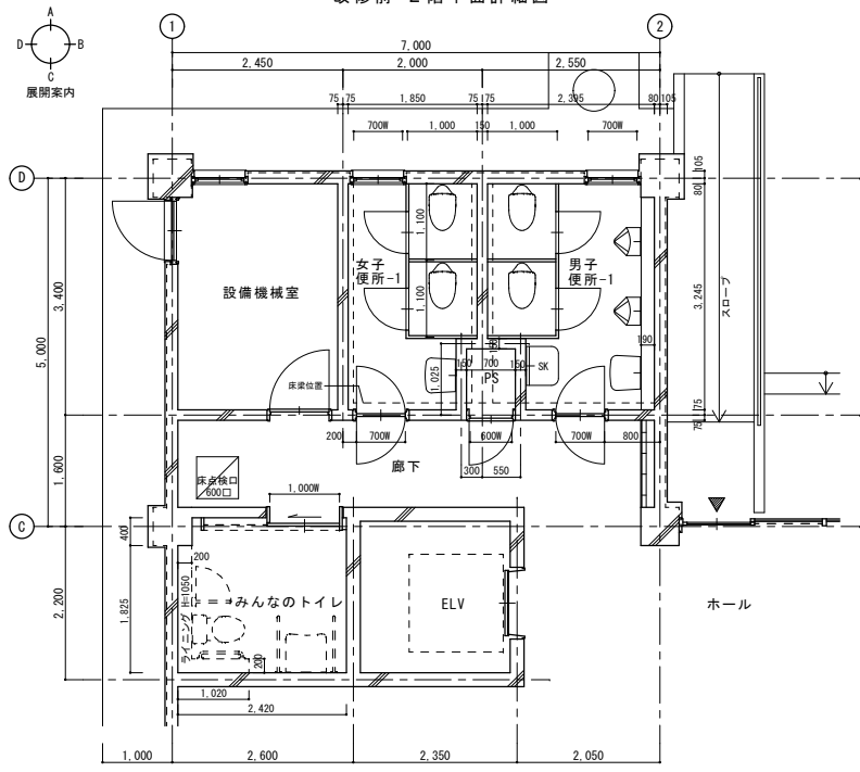
改修前 1階平面詳細図
