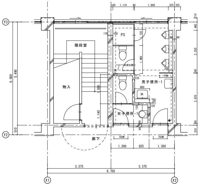
改修前 1階平面詳細図
