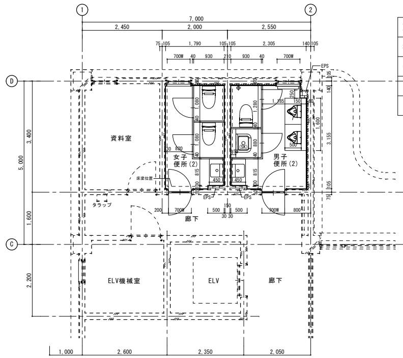
改修後 2階平面詳細図
