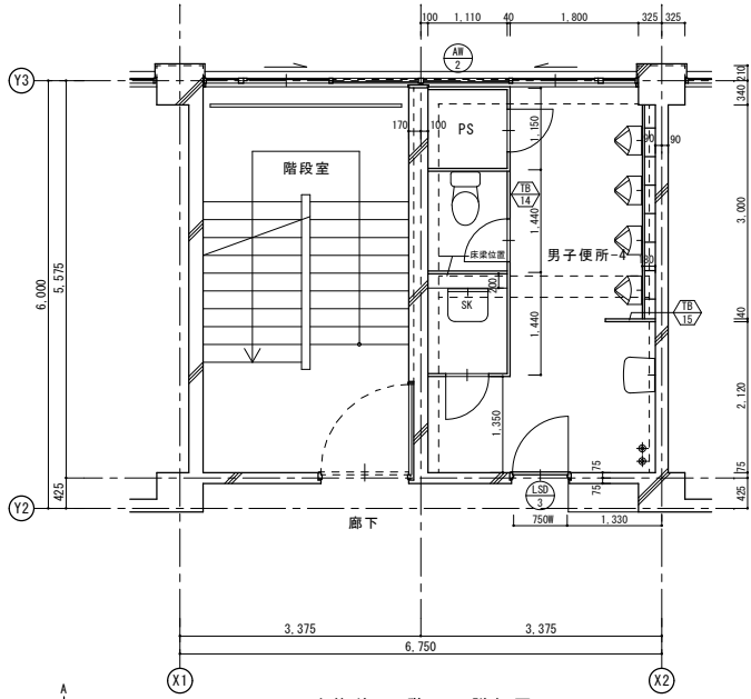
改修前 4階平面詳細図
