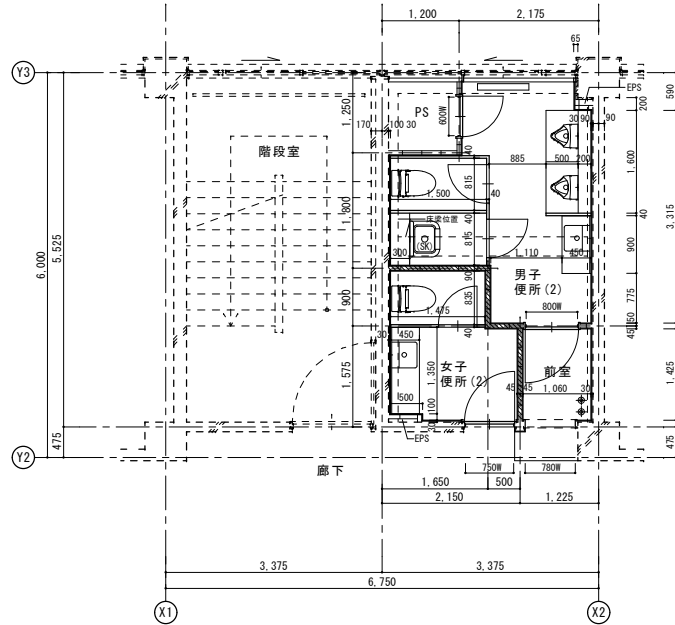
改修後 2階平面詳細図
