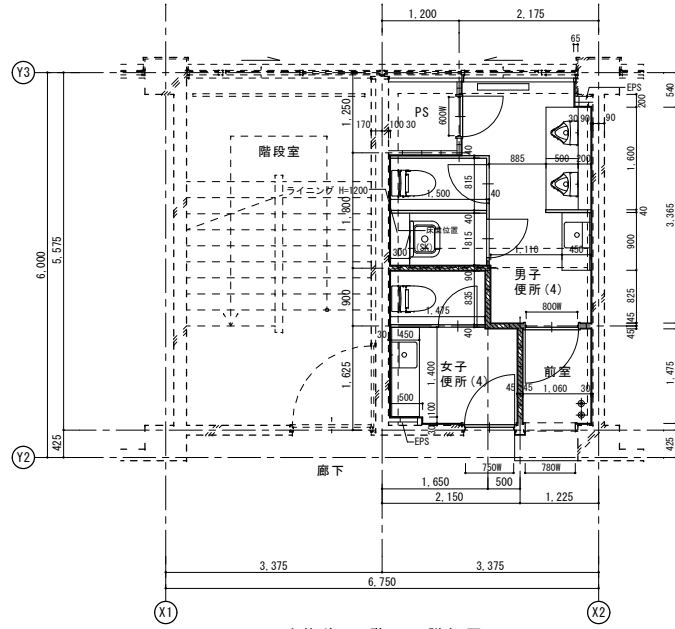
改修後 4階平面詳細図
