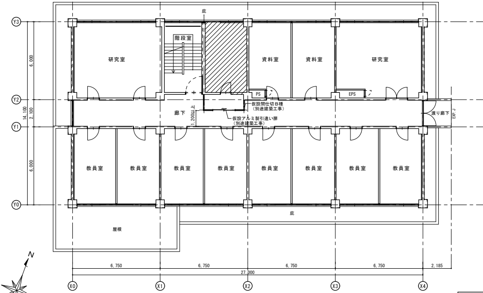
2階平面図
