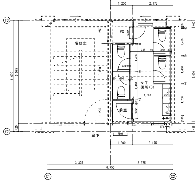
改修後 3階平面詳細図
