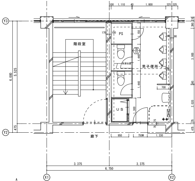
改修前 2階平面詳細図
