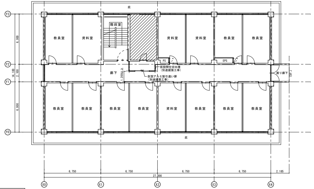
4階平面図
