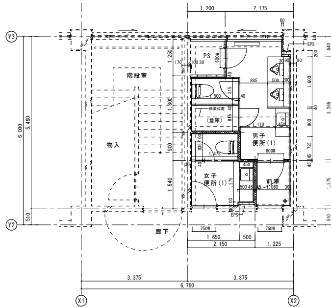
改修後 1階平面詳細図
