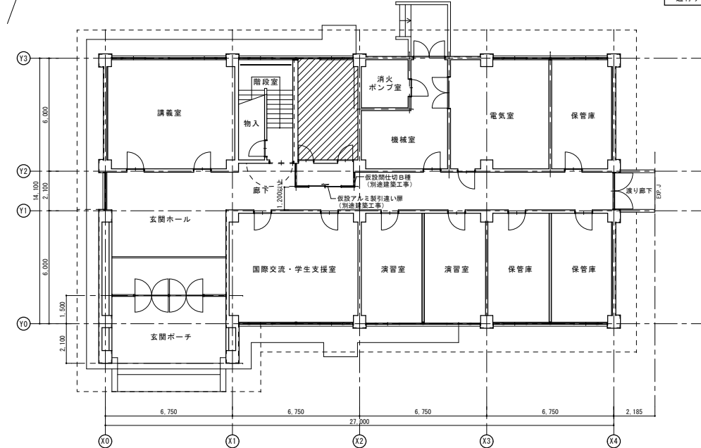
1階平面図
