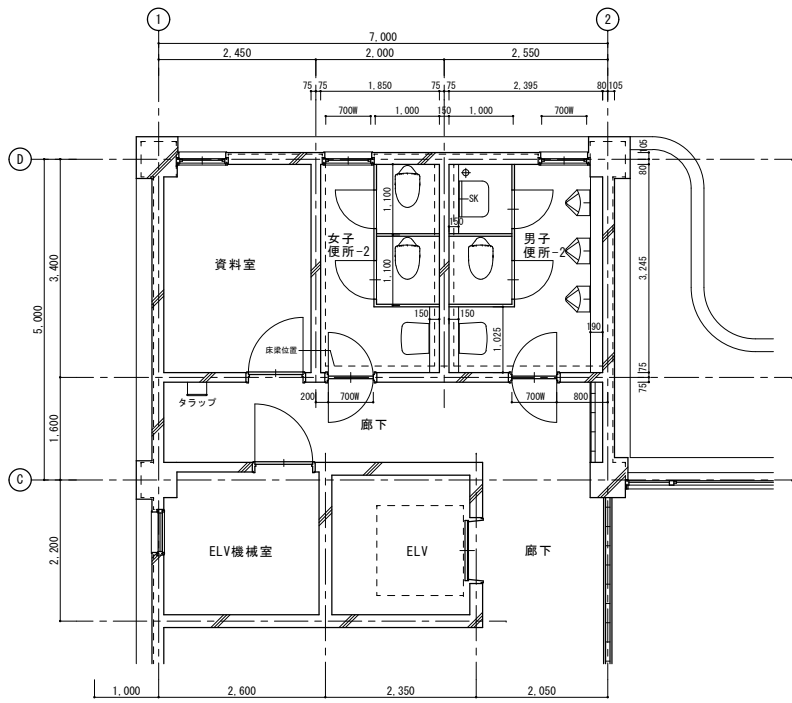
改修前 2階平面詳細図
