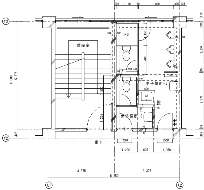
改修前 3階平面詳細図
