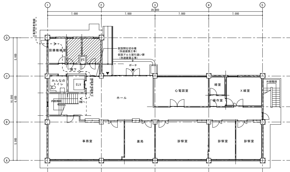
1階平面図
