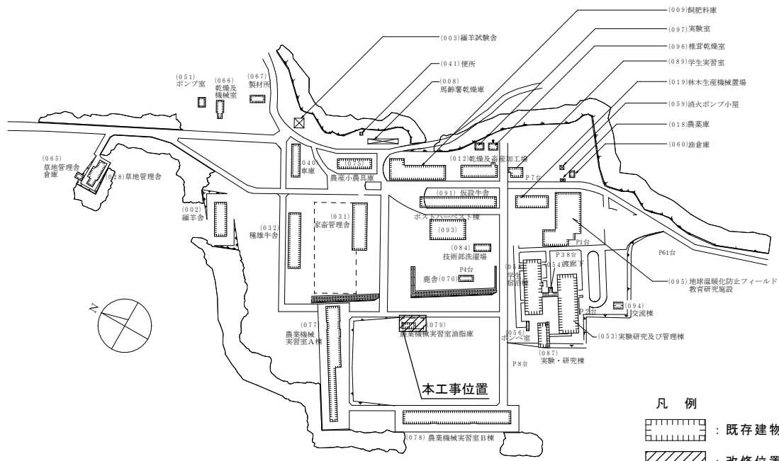
川渡2団地配置図 S=1/4000
