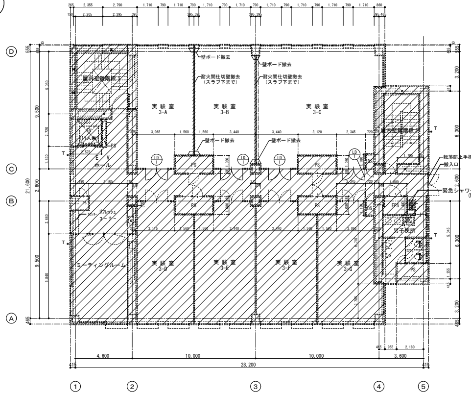
3階平面図（改修前） S=1/300
