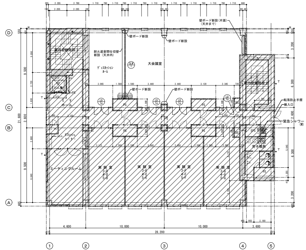
3階平面図（改修後） S=1/300
