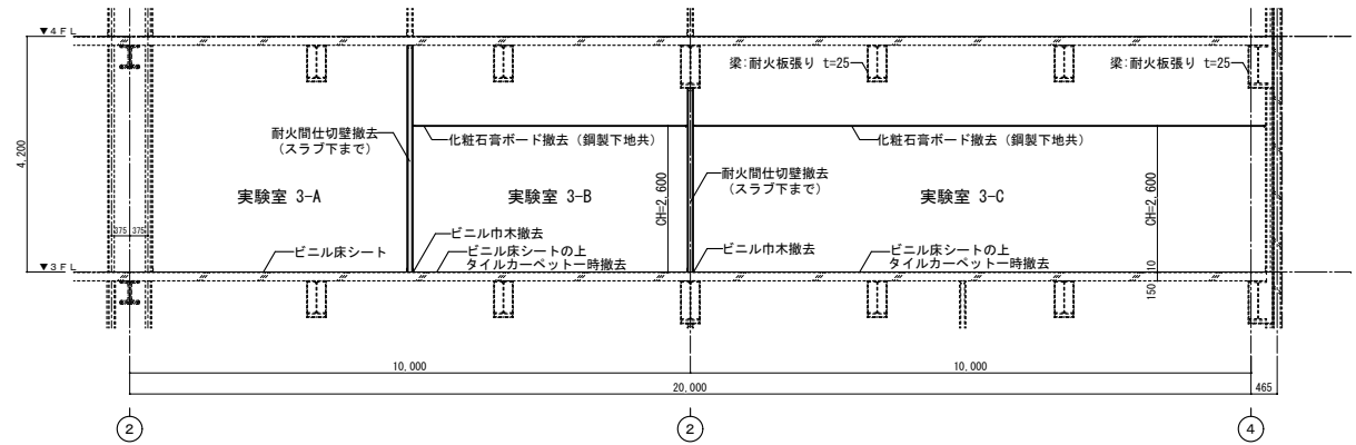
断面図-2 (改修前) S=1/150
