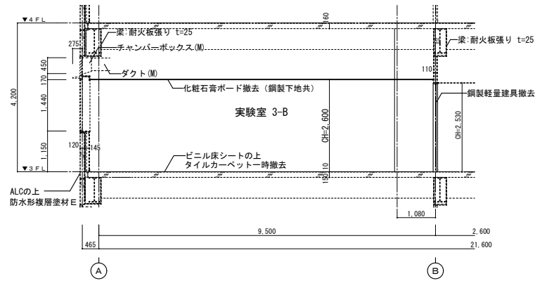
断面図-1 (改修前) S=1/150
