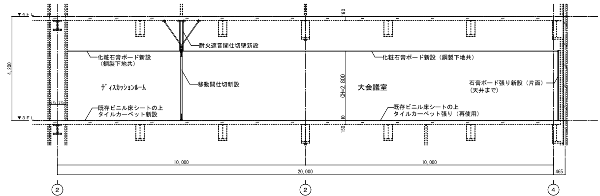
断面図-2 (改修後) S=1/150
