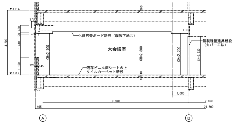
断面図-1 (改修後) S=1/150
