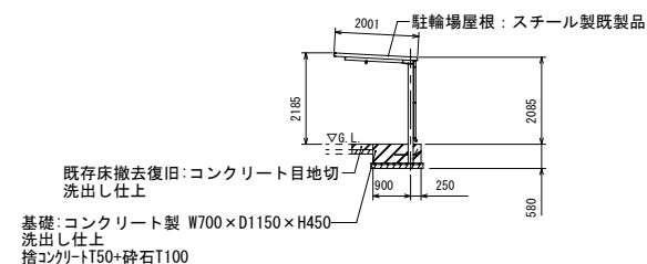
駐輪場14・15 断面図 2 S=1/200 (A4)
