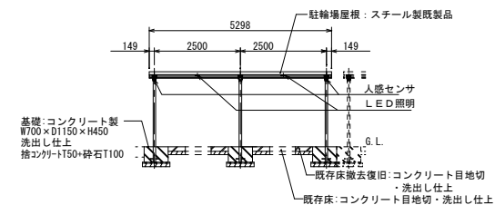
駐輪場1 断面図 1 S=1/200 (A4)
