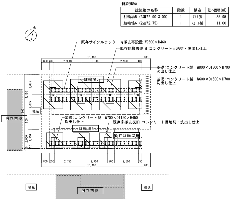
駐輪場5・6 平面詳細図 S=1/200 (A4)
