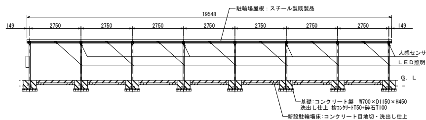
駐輪場4 断面図 1 S=1/200 (A4)
