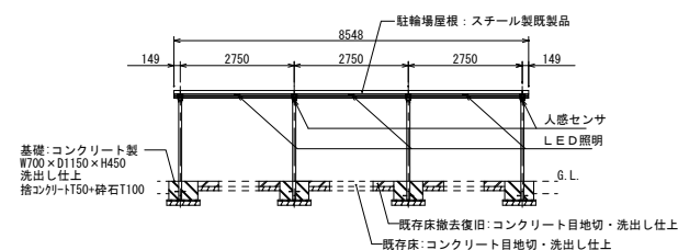
駐輪場2 断面図 1 S=1/200 (A4)
