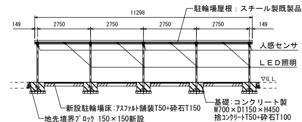
駐輪場14・15 断面図 1 S=1/200 (A4)
