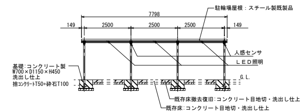
駐輪場3 断面図 1 S=1/200 (A4)
