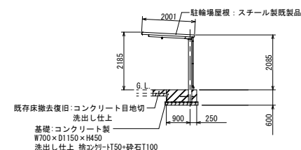
駐輪場1~4 断面図 2 S=1/200 (A4)
