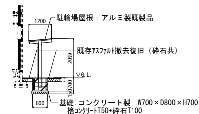
駐輪場9~13 断面図 2 S=1/200 (A4)
