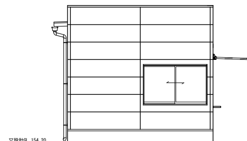
北側立面図 S=1:100
