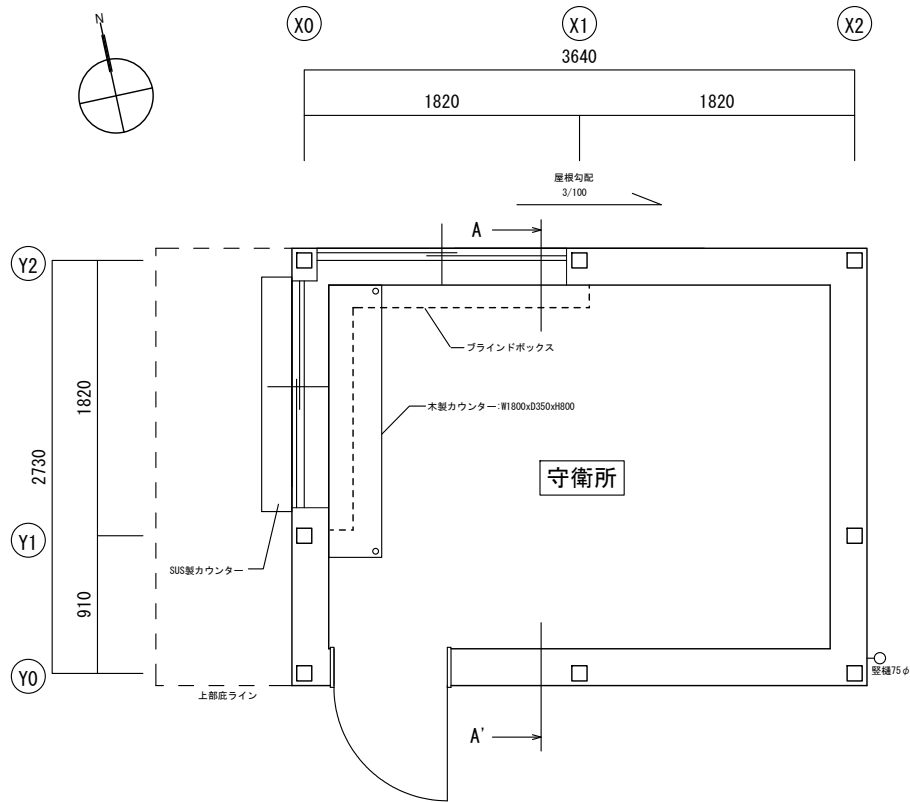
平面図 S=1/50
