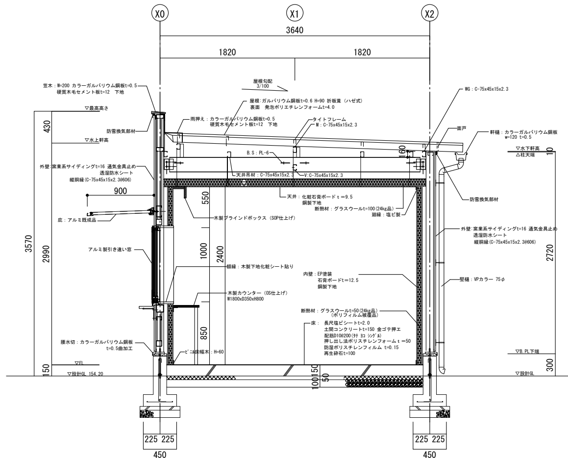
矩計図 S=1/50
