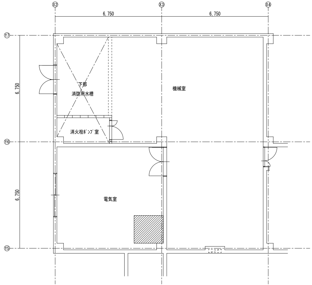
電気室平面図 S = 1 / 100
