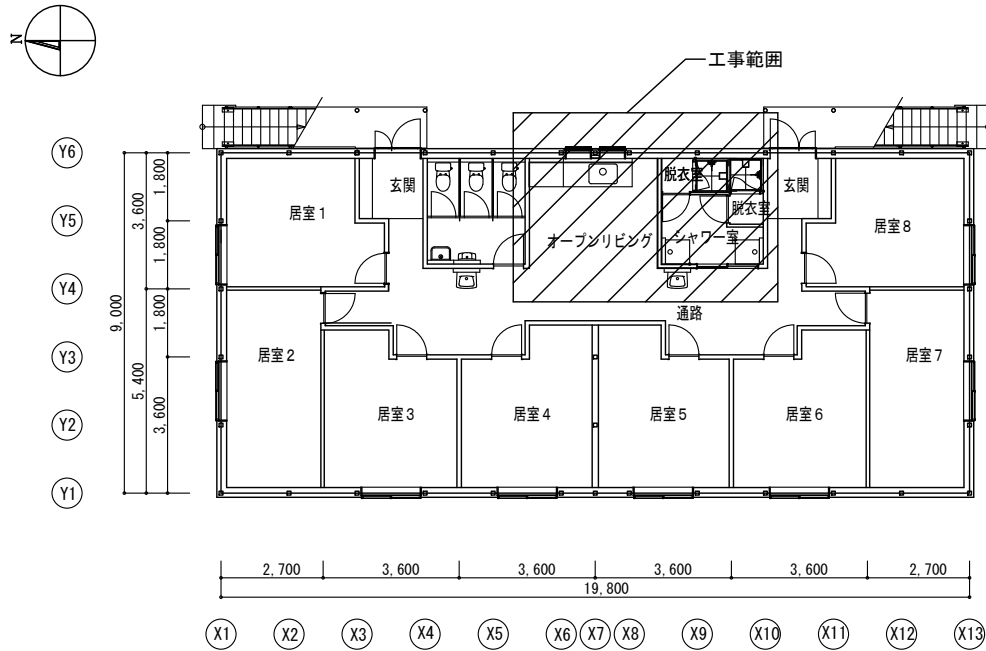
改修前平面図 1/200
