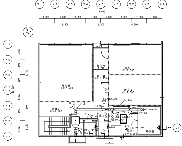
グローバルCOE研究棟2階平面図（改修後）
