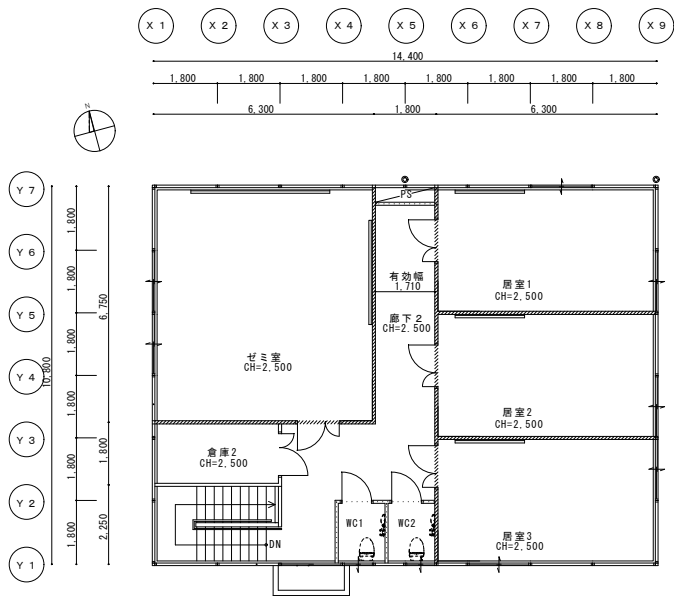
グローバルCOE研究棟2階平面図（改修前）
