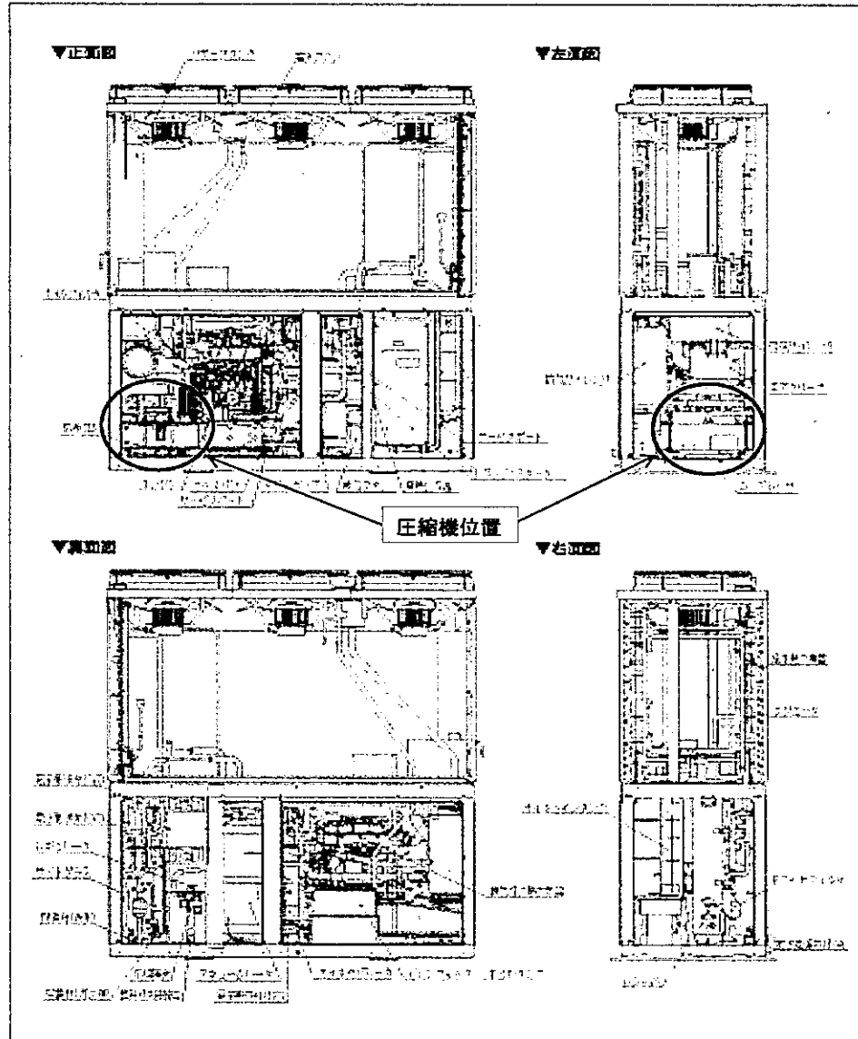
図1.8/構造図 [450形]
