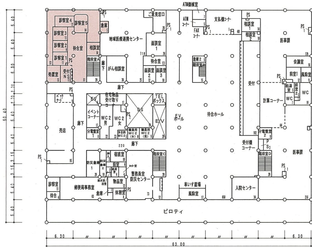
外来診療棟A 改修前1階平面図 2,747㎡
