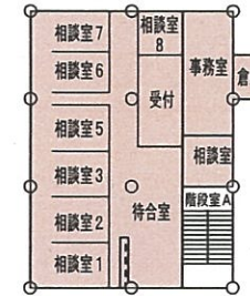
工事範囲 改修後1階平面図 200㎡
