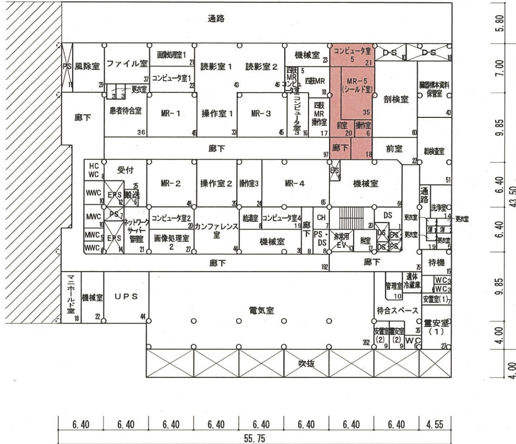
東病棟 改修地下1階平面図 2,487 m 2
