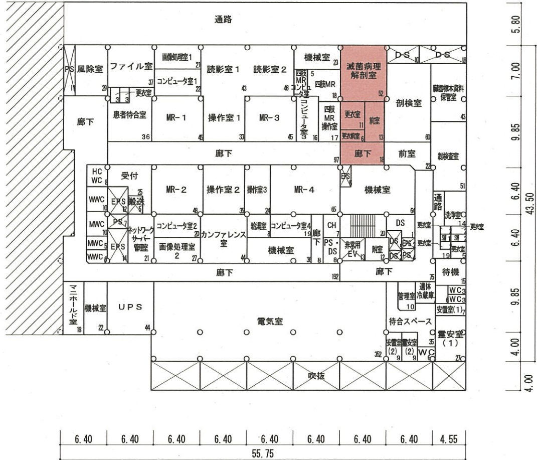
東病棟 既存地下1階平面図 2,487 m ²
