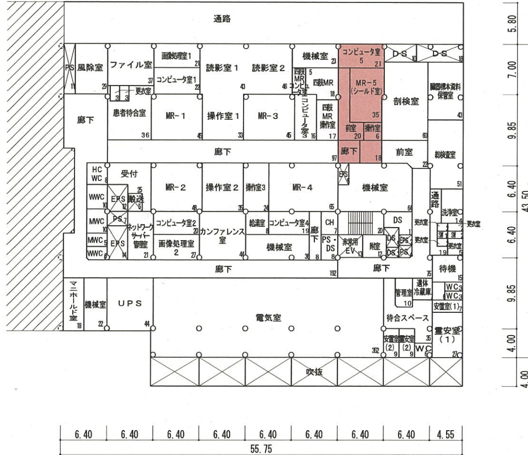
東病棟 改修地下1階平面図 2,487㎡
